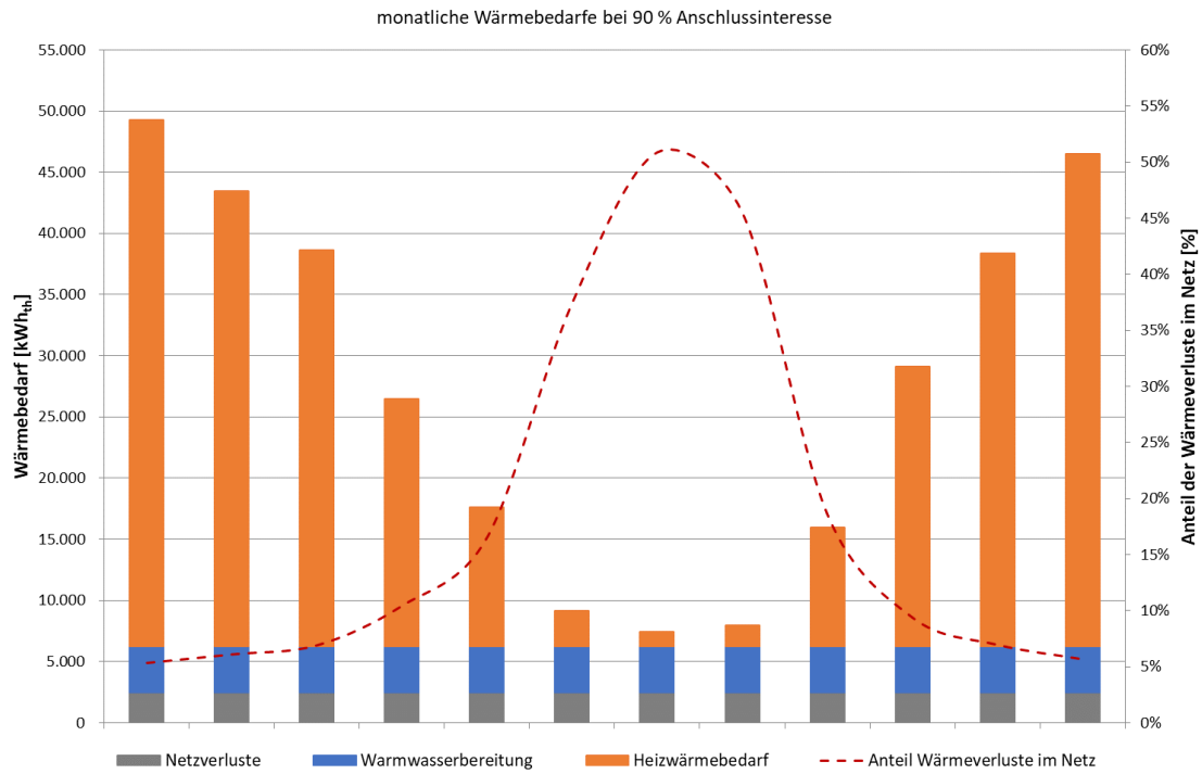
Abbildung 38: monatlicher Wärmebedarf Fall 1: 90 % Anschlussdichte
