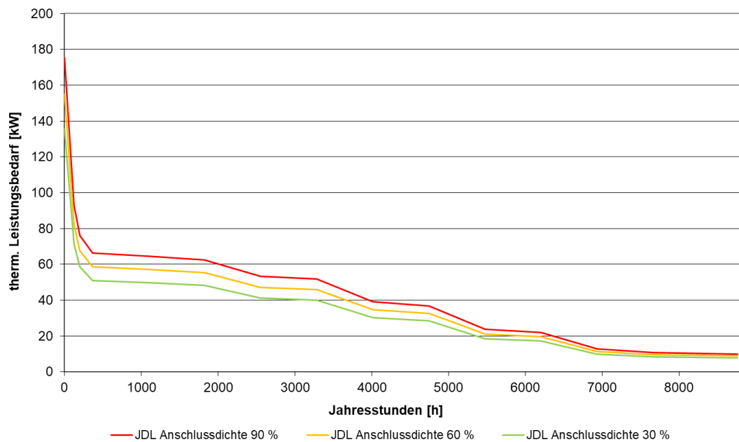
Abbildung 41: thermische Jahresdauerlinie für den Fall 1,2 und 3
