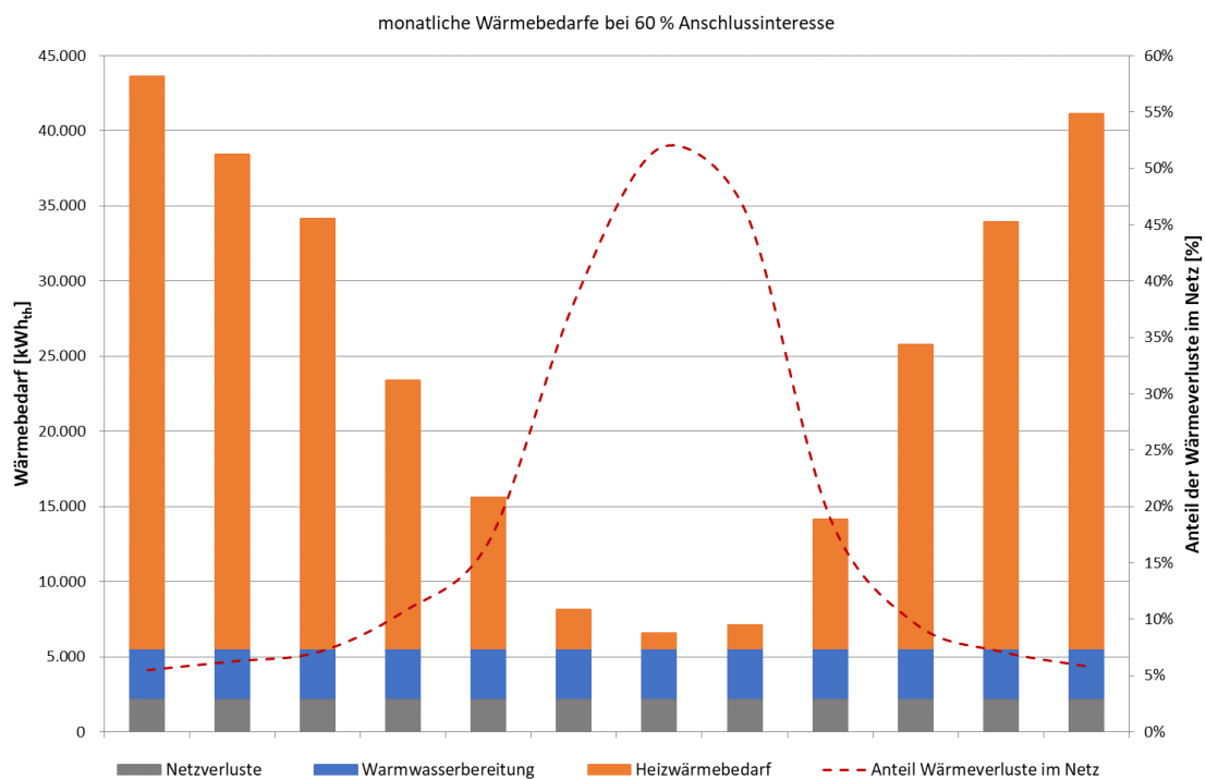
Abbildung 39: monatlicher Wärmebedarf Fall 2: 60 % Anschlussdichte
