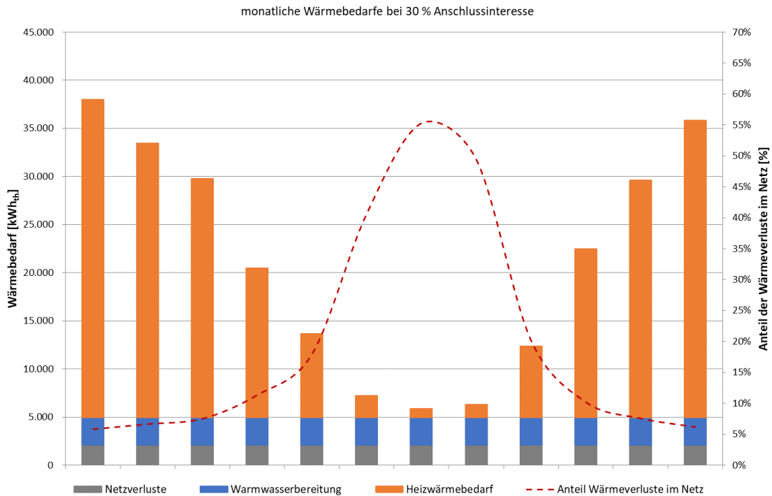
Abbildung 40: monatlicher Wärmebedarf Fall 3: 30 % Anschlussdichte
